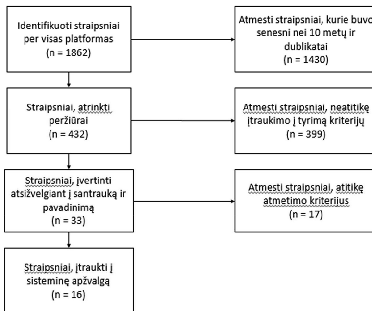
1 pav. Mokslinių straipsnių atrankos schema
