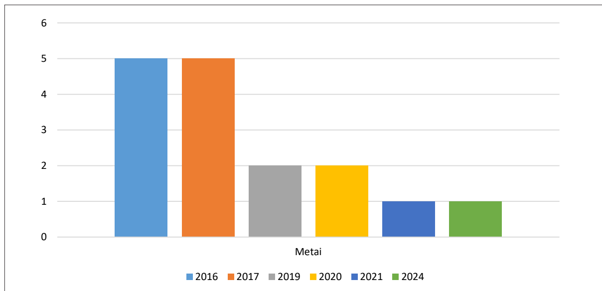
2 pav. Į sisteminę literatūros apžvalgą įtrauktų straipsnių publikavimo metai (vnt.)
