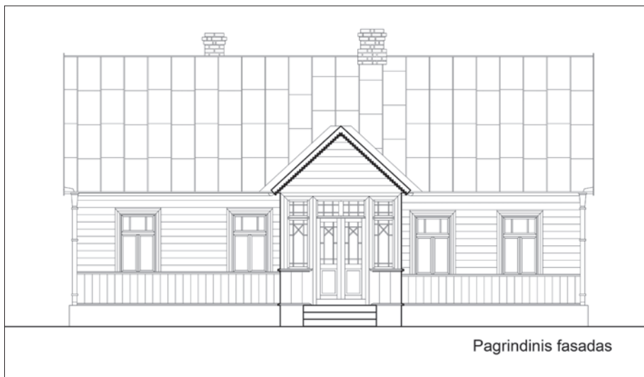
7 il. Petrusevičių namo apmatavimo brėžinys, 2023 m.
